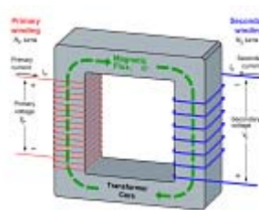
transformer 变压器 [biàn yā qì]
