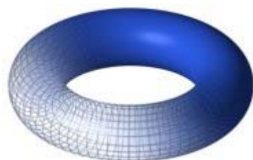
torus
