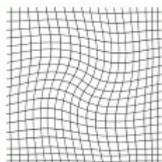
net
