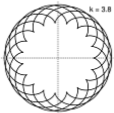
epicycloid 外摆线
