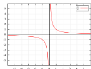
hyperbola
