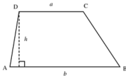
trapezoid 梯形
